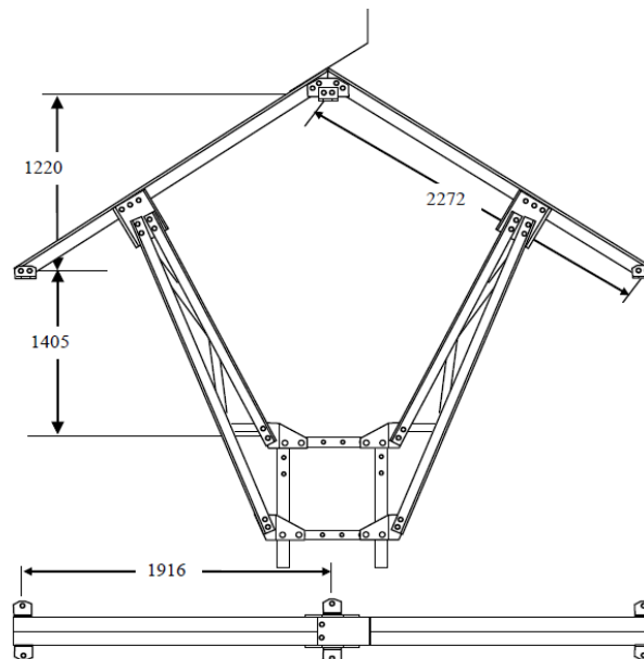
Detalle cruceta bóveda de celosía antiposada `CBCA`
