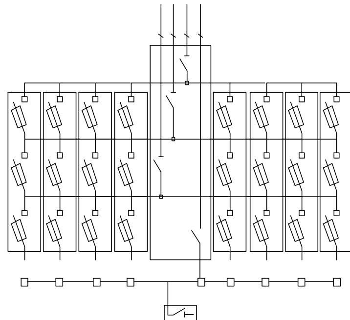
ESQUEMA ELECTRICO
