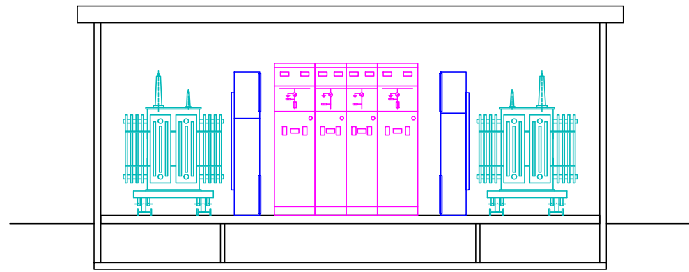
SECCIÓN TRANSVERSAL
