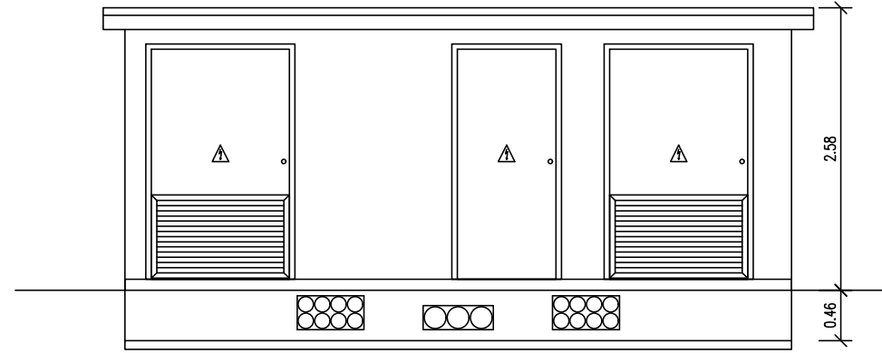
ALZADO FRONTAL
