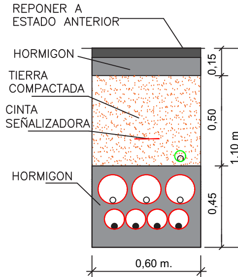
SECCIÓN CANALIZACIÓN E_1:20
