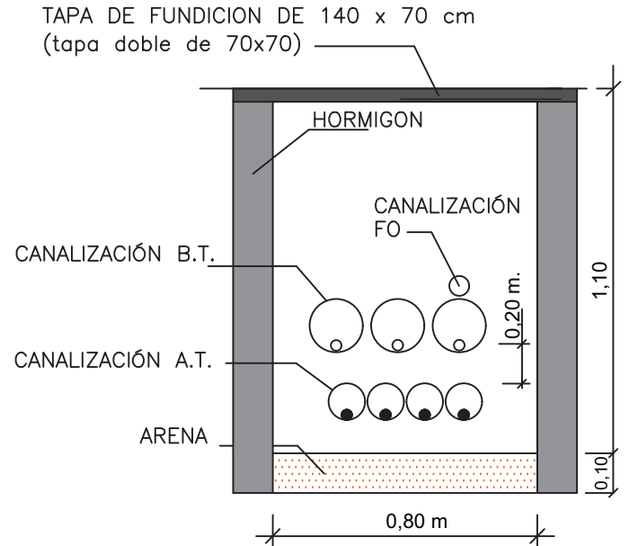
SECCIÓN ARQUETAS BAJA Y MEDIA TENSION E_1:20
